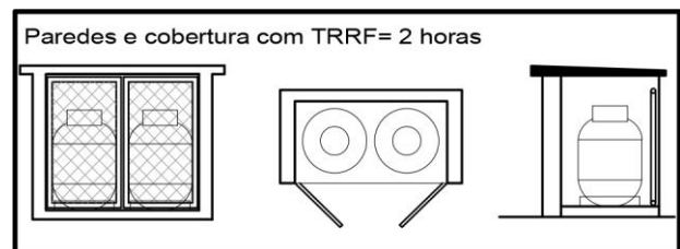
Figura 1– Central com recipientes de 190 Kg de GLP
