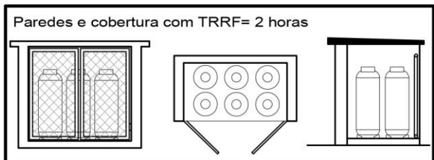
Figura 2– Central com recipientes de 45 Kg de GLP
