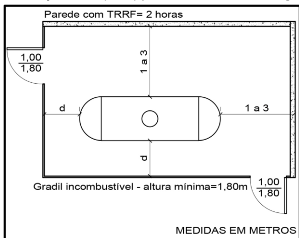
Figura 7 - Central de GLP com recipiente estacionário e construção de 02 (duas) paredes resistentes ao fogo
